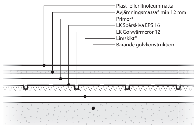
LK EPS 16 limmat mot bärande golv i våta utrymmen. Ytskikt plast- eller linoleummatta
